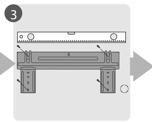
3 Закрепите монтажную пластину
